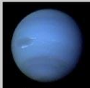
Нептун
