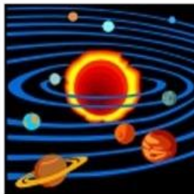
солнечная система
