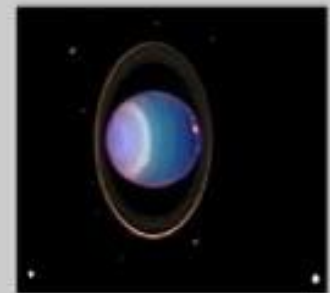
Уран
