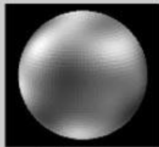
Плутон
