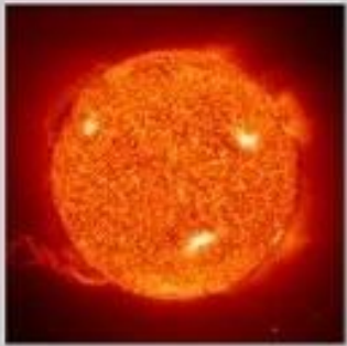
Солнце
